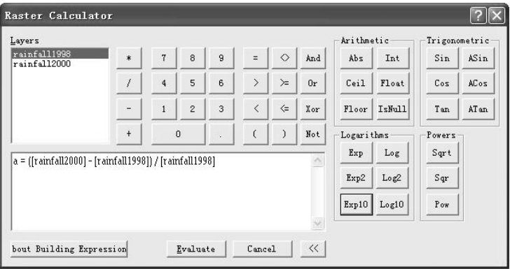
图 8.67 栅格计算器的数学算术运算
