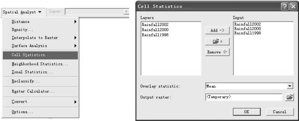
图 8.52 单元统计的操作过程
