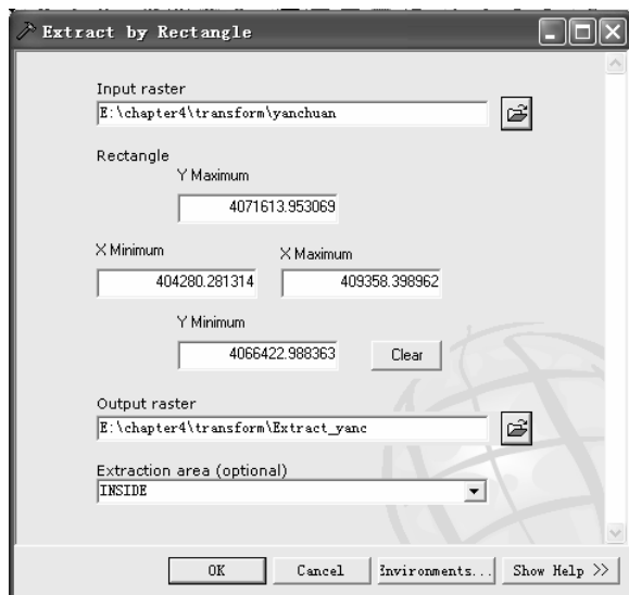
图 4.33 Extract by Rectangle 对话框
