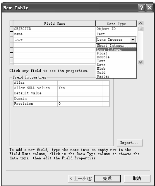
图 3.34 属性字段编辑对话框
